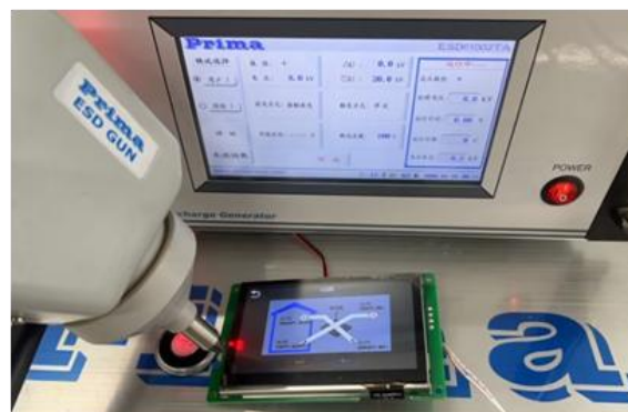
图 4-2 ESD 测试图
