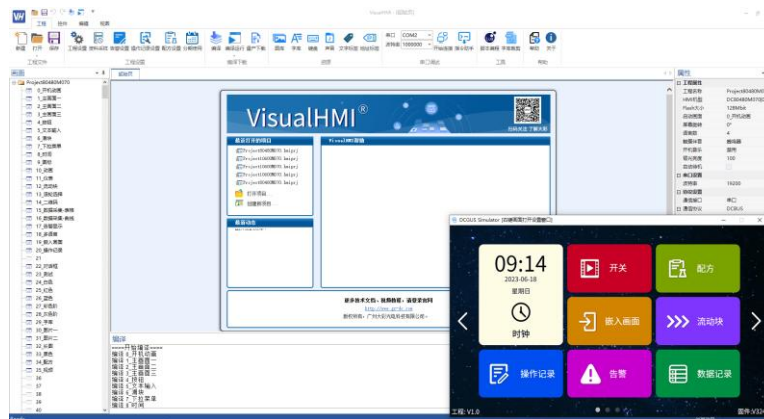
图 6-1 VisualHMI 主界面
